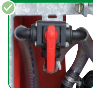
Hahn Spritzen/Spülen
